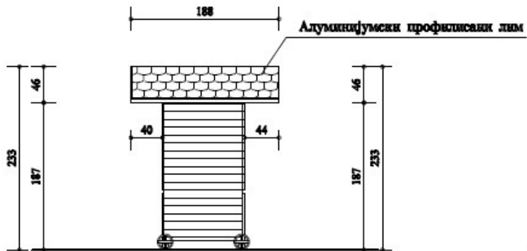
БОЧНИ ИЗГЛЕД
