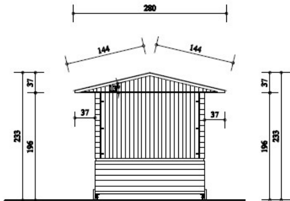
ПРЕДЊИ ИЗГЛЕД
